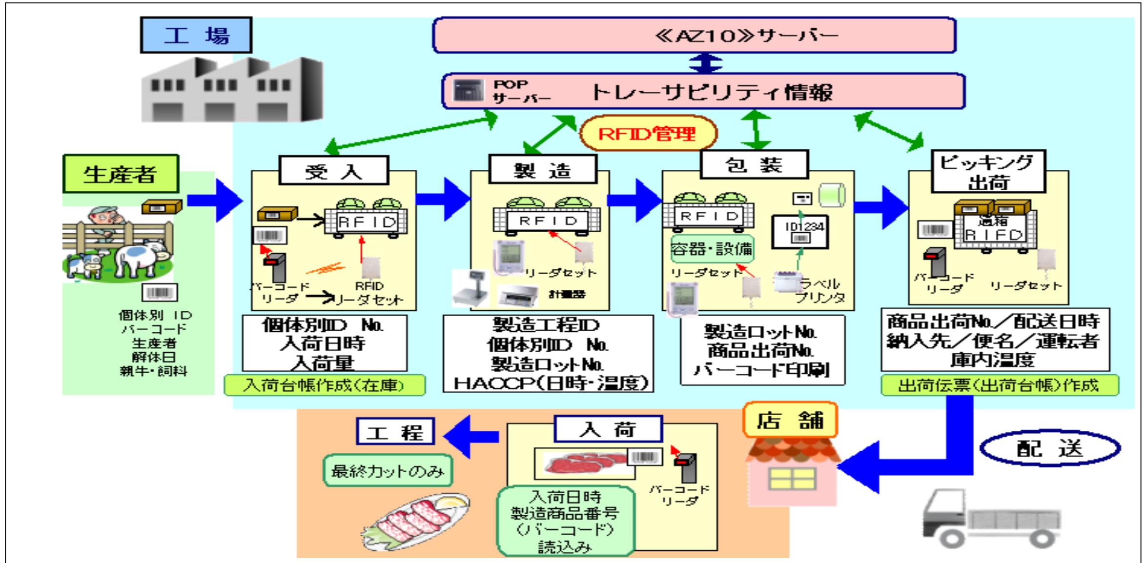
図13：食品工場のRFIDを使ったトレーサビリティシステム
