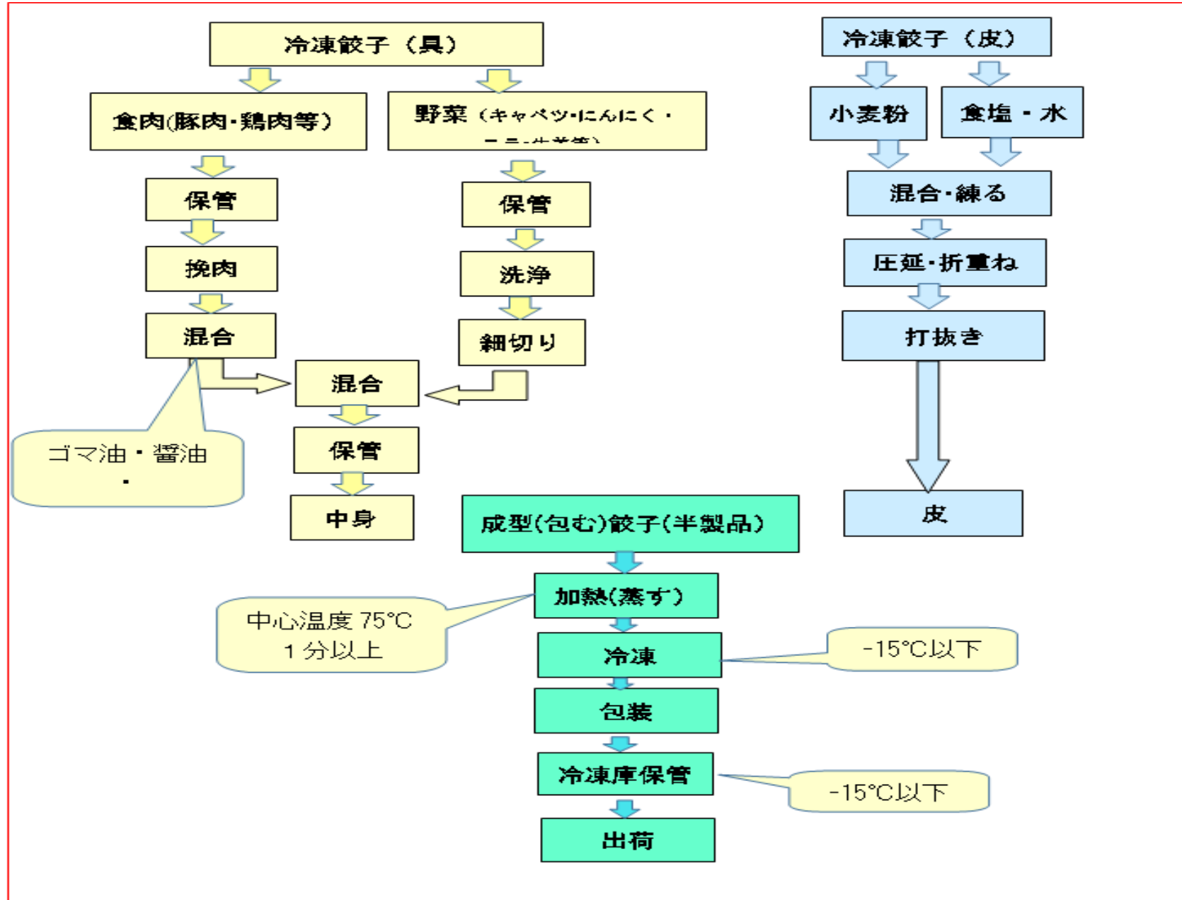
図15：フローチャート（冷凍餃子）
